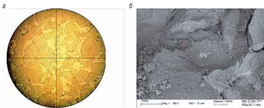
Рис. 4. Фосфатные породы, вскрытые в скважине LL-106:
