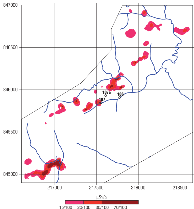
Рис. 3. Карта гамма-аномалий сектора Ранчо-Чири (аномалии с МЭД фотонного излучения более 0,15 мк 3 )
