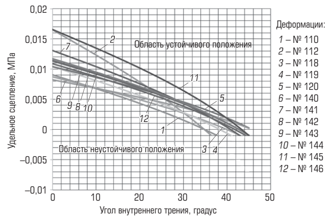
Рис. 2. Зависимость между углом внутреннего трения и удельным сцеплением в фенитах прибортового породного массива карьера рудника «Железный»
