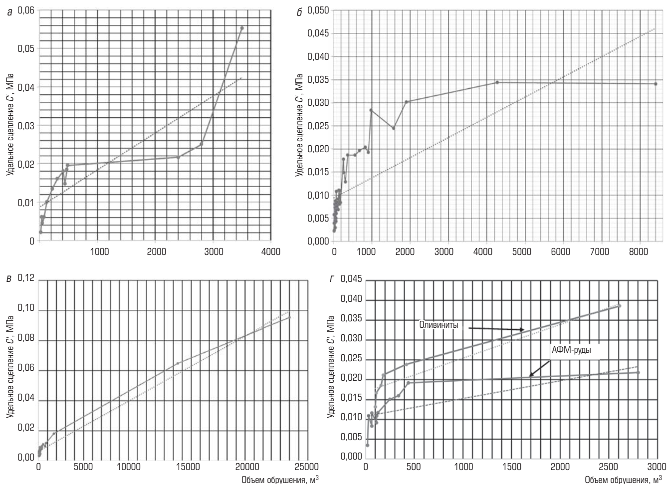
Рис. 3. Изменение удельного сцепления в пироксенитах (а), ийолитах (б), фенитах (в), оливинитах и АФМ-рудах (г) по мере увеличения объема обрушения (пунктиром показана линия тренда)
