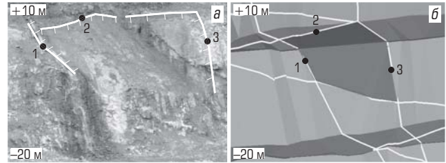
Рис. 1. Фото обрушения в уступе (а) и его реконструированная трехмерная модель (б)
