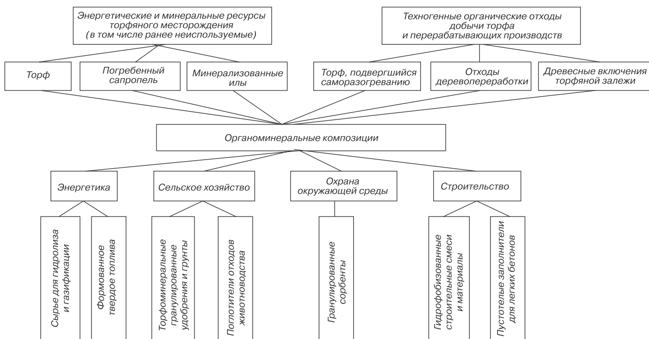
Рис. 1. Принципиальная схема использования ресурсов торфяных месторождений, отходов добычи и переработки
