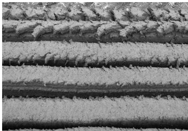
Рис. 3. Свежесформованная торфяная лента с признаками нарушения целостности куска (кольцевое «ершение»)
