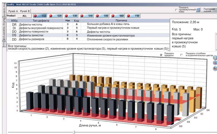
Система контроля качества Simetal Quality Expert
